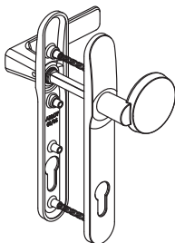
Palière extérieure sur plaque pour barreur ABLOY Entraxe 92 mm (compatible avec serrures EL/MP motorisées et mécaniques)
