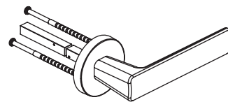
Béquille extérieure sur rosace pour barreur ABLOY Entraxe 70 ou 72 mm (compatible avec serrures EL/MP électriques)
