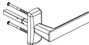
Béquille extérieure sur rosace pour barreur ABLOY Entraxe 92 mm (compatible avec serrures EL/MP électriques)
