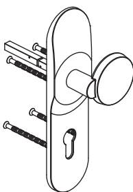
Palière extérieure sur plaque pour barreur ABLOY Entraxe 70 ou 72 mm (compatible avec serrures EL/MP motorisées et mécaniques)
