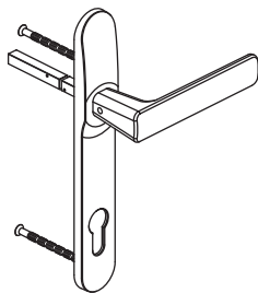
Béquille extérieure sur plaque pour barreur ABLOY Entraxe 92 mm (compatible avec serrures EL/MP électriques)
