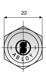
Sylinterin etupinta
