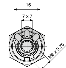
Sylinterin takaosa
