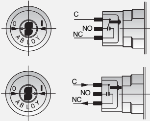
KYTKENTÄKAAVIO
